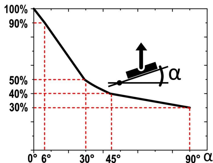
Chiffres indiquant la capacité de charge selon la direction pour le TML 90 R
