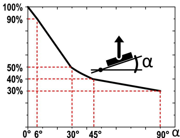
Cifras de capacidad de carga dependientes de la dirección para el TML 90 R
