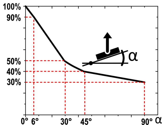
Richtungsabhängige Traglastzahlen für den TML 90 R
