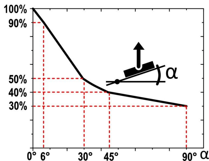
Løftekapasitetsendringer ved vinkling av lasten. TML 90 R
